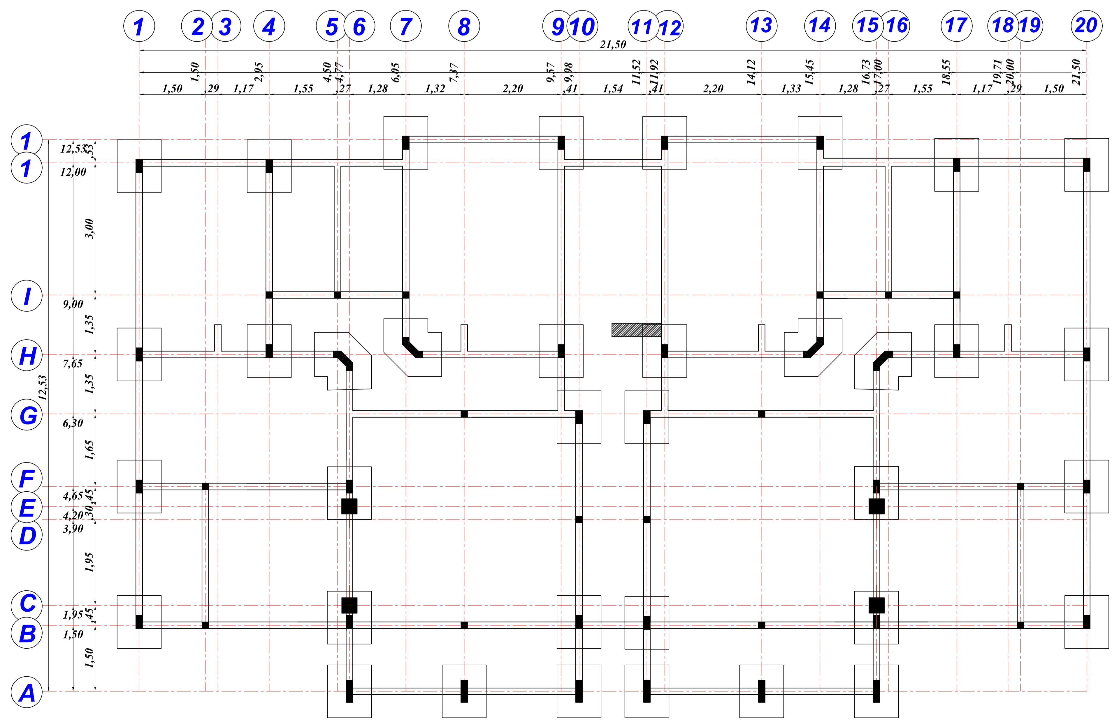
IMMEUBLE R + 1 ( FONDATIONS )
