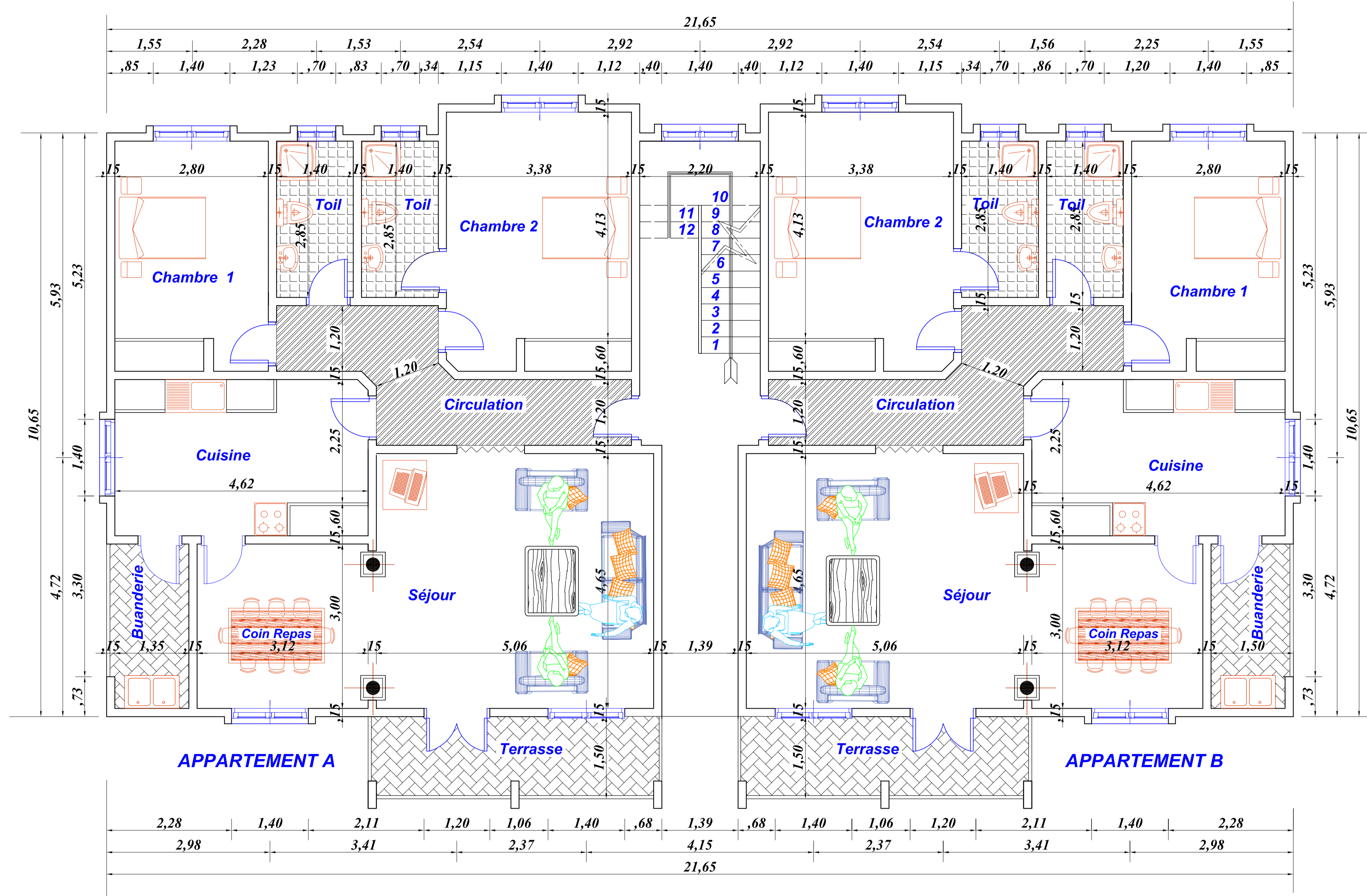
IMMEUBLE R + 1 ( REZ DE CHAUSSEE )
