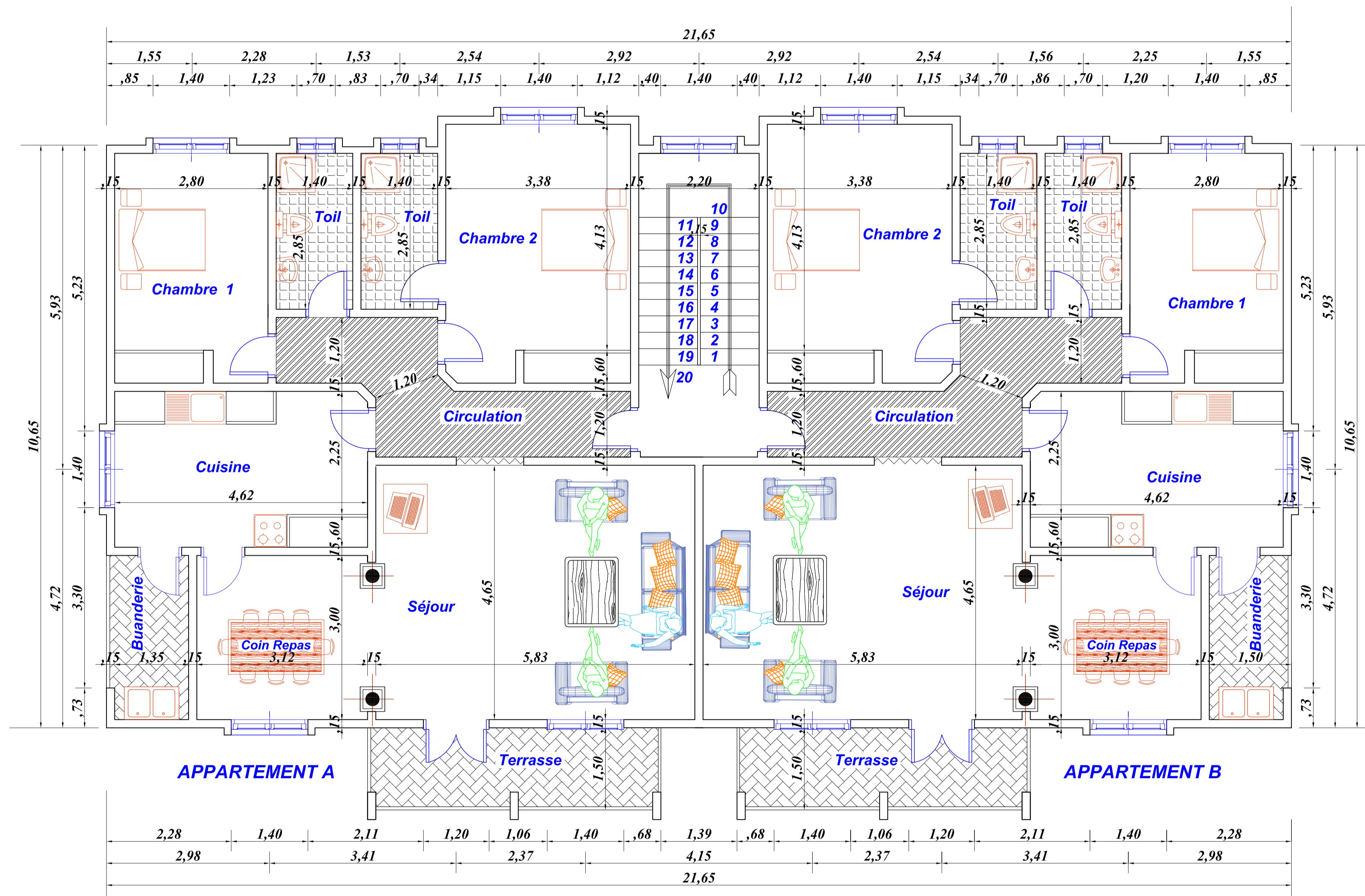
IMMEUBLE R + 1 ( ETAGE 1 )
